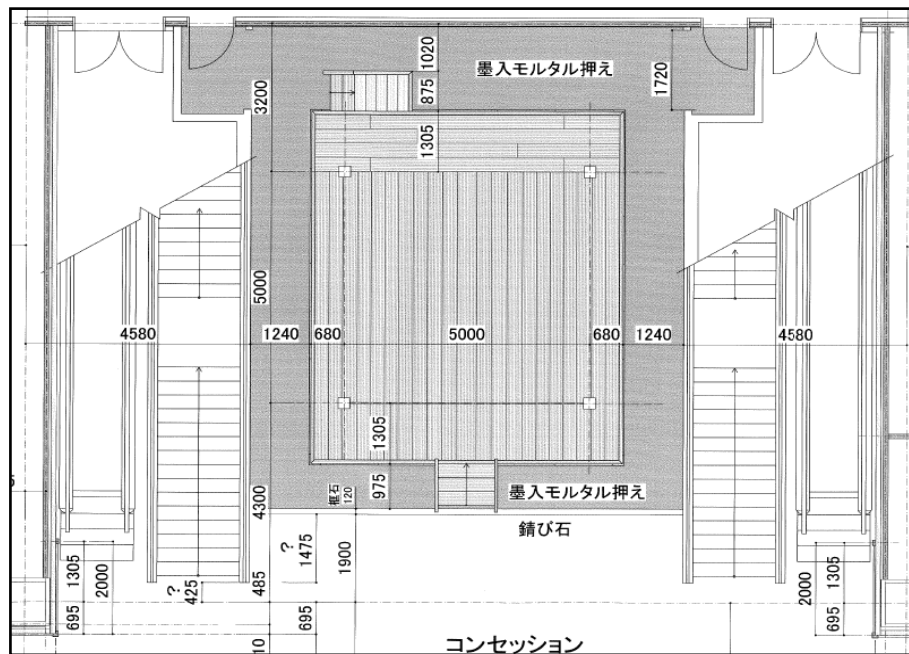
江戸舞台平面図
