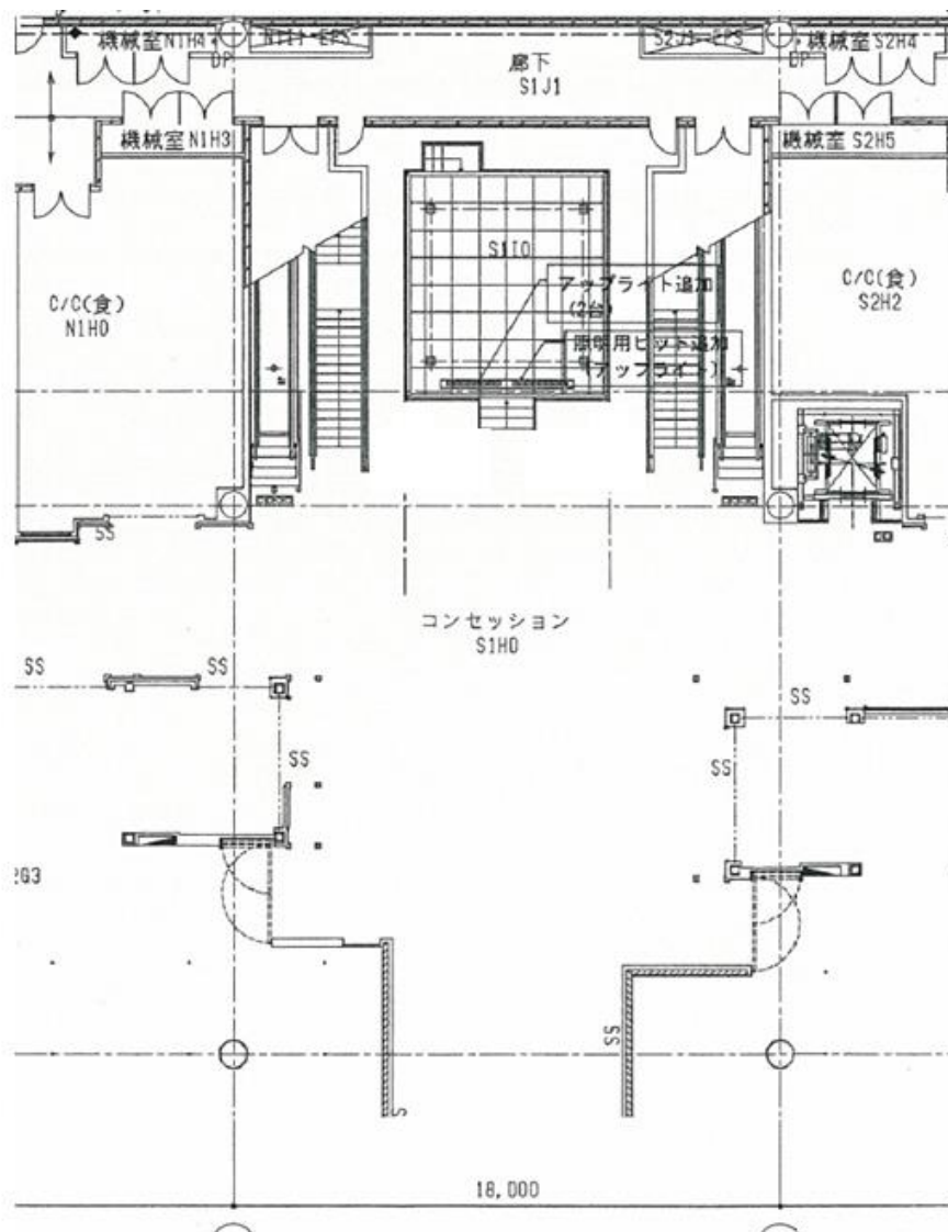
江戸舞台周辺前 平面図
